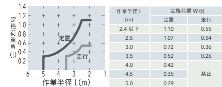
ViO45-6Aクイックヒッチ仕様(標準アーム0.14m 2 バケット付き)
