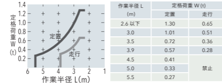
ViO55-6Aクイックヒッチ仕様(標準アーム0.16m 2 バケット付き)
