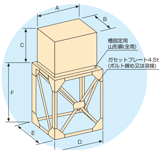
〔備考〕槽の固定方法、補強鋼材方法等は、一例を示す。
