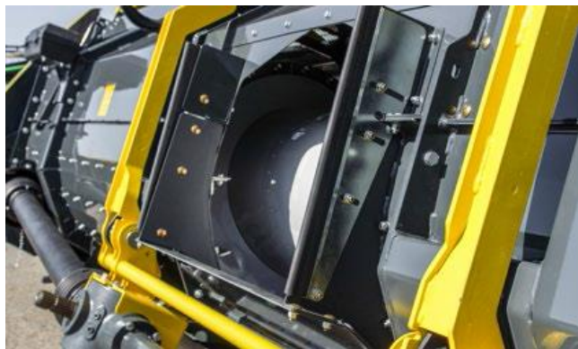
アダプターを使用すれば自走ハーベスターの型式に合わせて間口変更可
