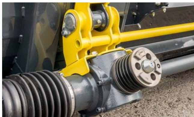
マルチカプラ(左)とオートカップリング(右)で簡単マッチング
