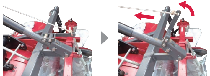
サイド整形板付きソリフリー状態
