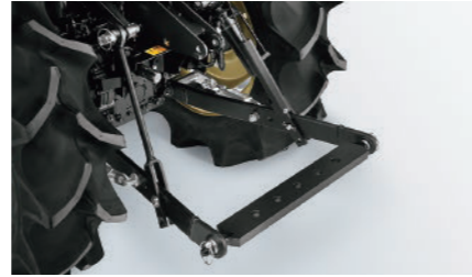
リンケージドロバ ロアリンクに装着できるドロバヒッチです。
