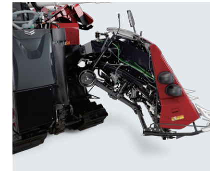
5 刈取サイドオープン (キャストレス)
