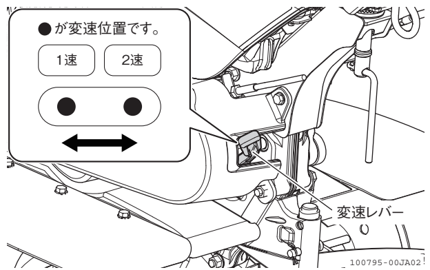
図 2-24 変速レバー
