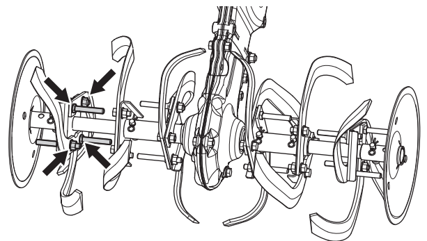
図 4-30 耕うん爪取付ボルト
