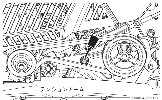
図 4-4 テンションアーム支点
