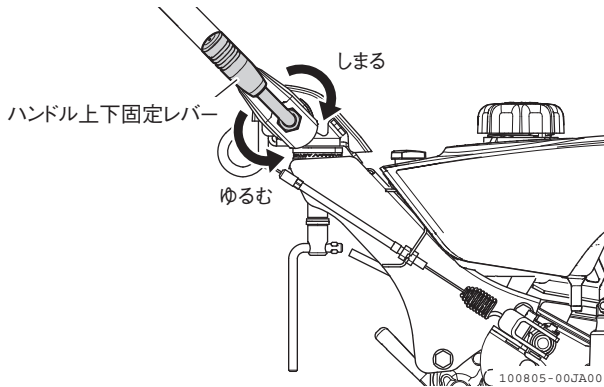
図 2-5 ハンドル上下固定レバー
