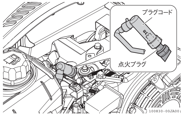
図 4-36 点火プラグ・プラグコード
