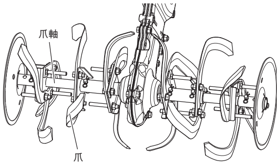
図 4-1 爪と爪軸
