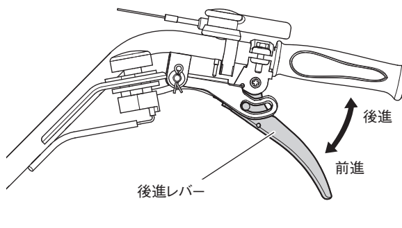
図 2-4 後進（握るとバック）レバー（-B、-D、-S型式）
