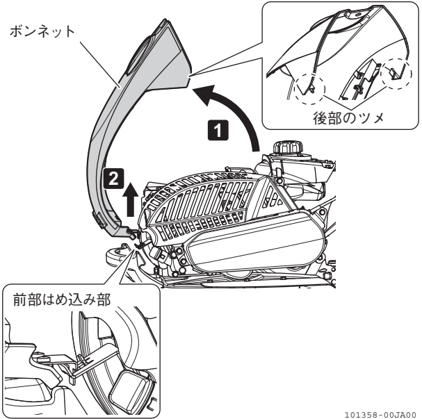
図 4-35 ボンネット
