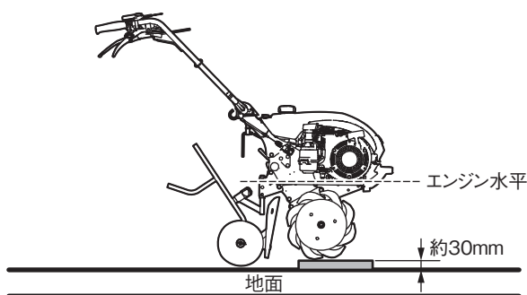
図 4-14 オイル点検・交換時の水平状態
