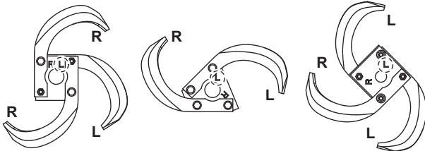
図 4-33 爪交換
