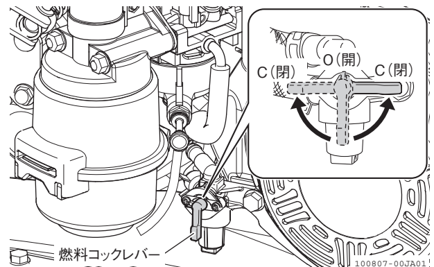
図 2-27 燃料コックレバー
