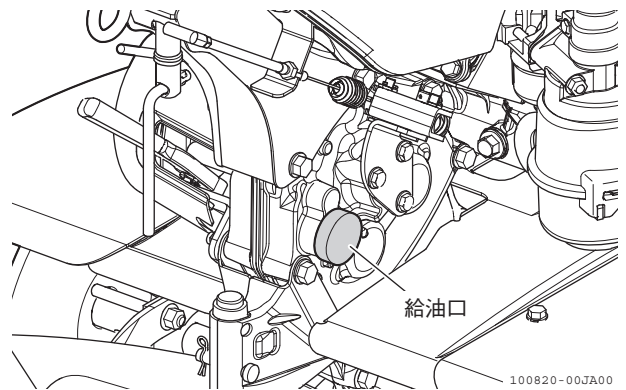
図 4-17 走行ミッションの給油口
