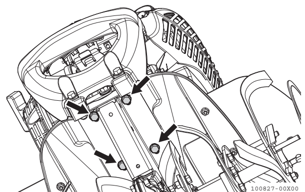
図 4-31 エンジン取付ボルト
