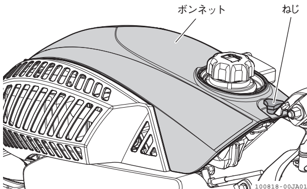
図 4-34 ボンネット
