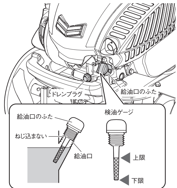
図 4-15 点検のしかた
