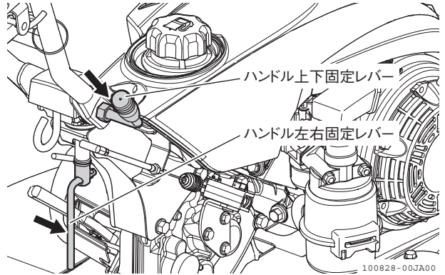
図 4-29 ハンドル上下固定レバー・ハンドル左右固定レバー
