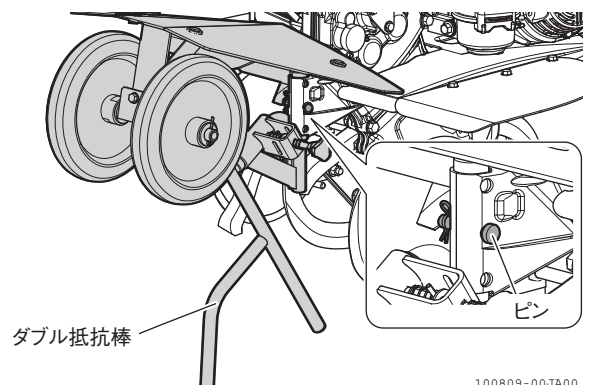
図 2-12 ダブル抵抗棒 (-D型式)
