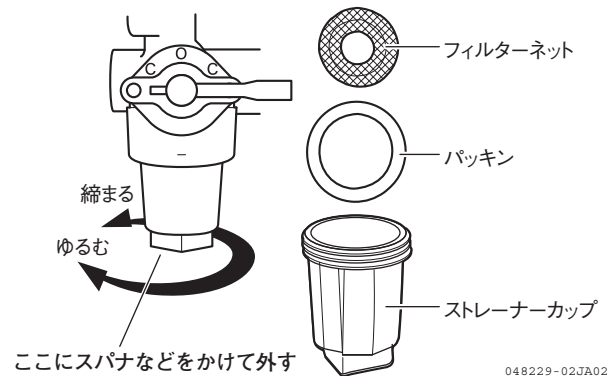
図 4-22 燃料コシ器
