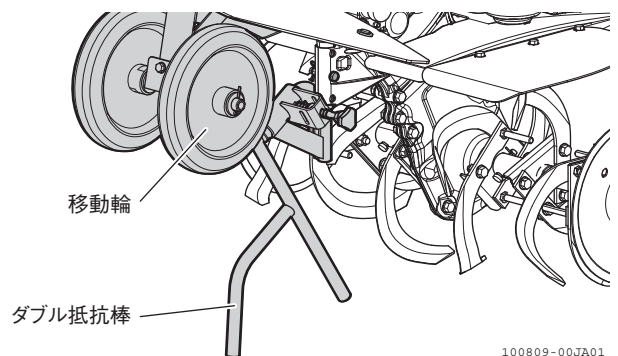
図 2-8 回転式移動輪 (-D型式)
