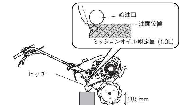
図 4-17 走行ミッションの給油口
