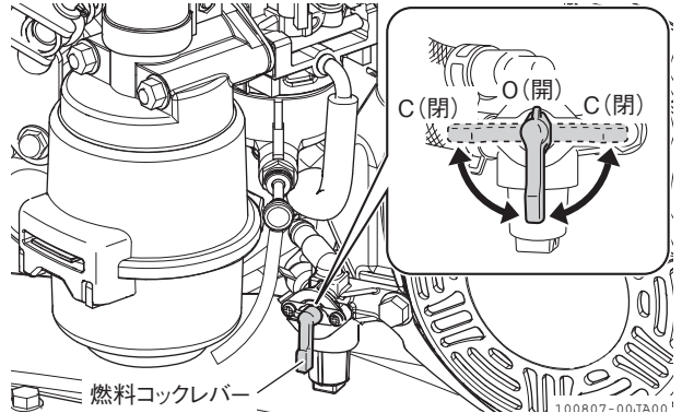
図 2-15 燃料コックレバー
