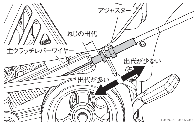
図4-26 主クラッチレバーアジャスターの調整
