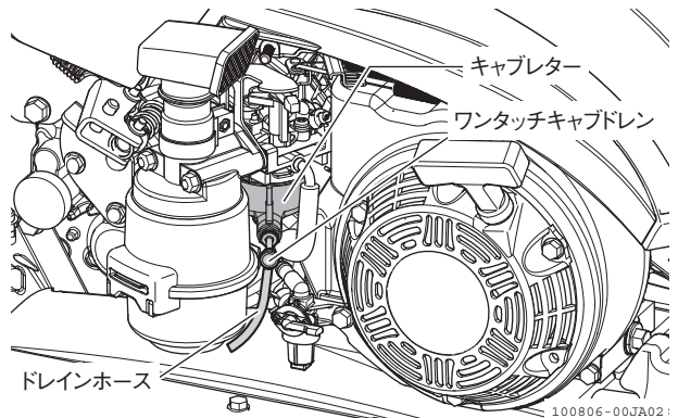
図 2-16 ワンタッチキャブドレン
