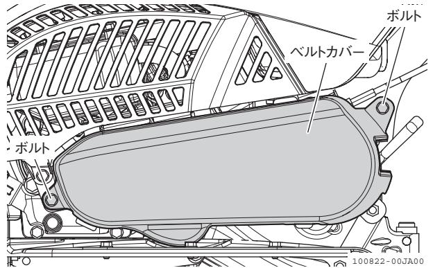
図 4-23 ベルトカバー
