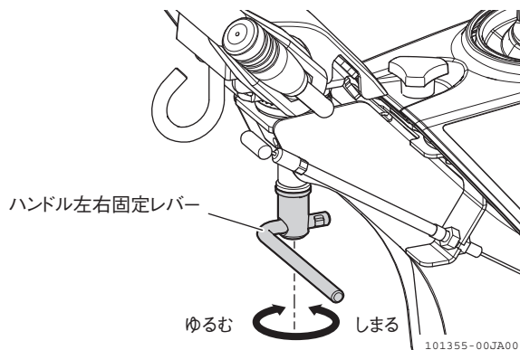
図 2-6 ハンドル左右固定レバー (-D型式)
