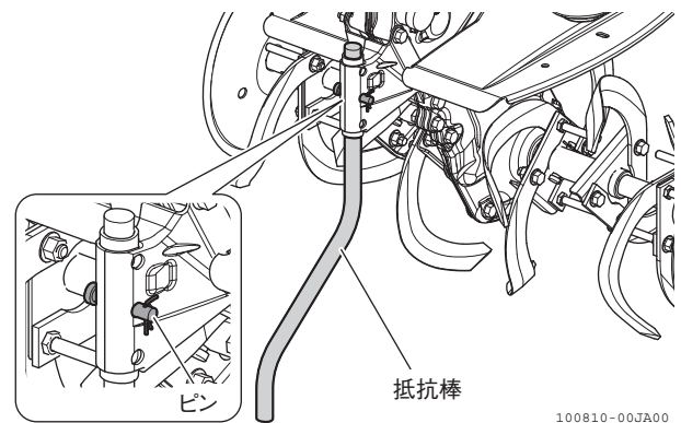
図 2-11 抵抗棒 (-D型式以外)
