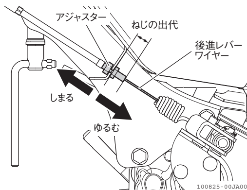
図 4-28 後進レバーの調整のしかた
