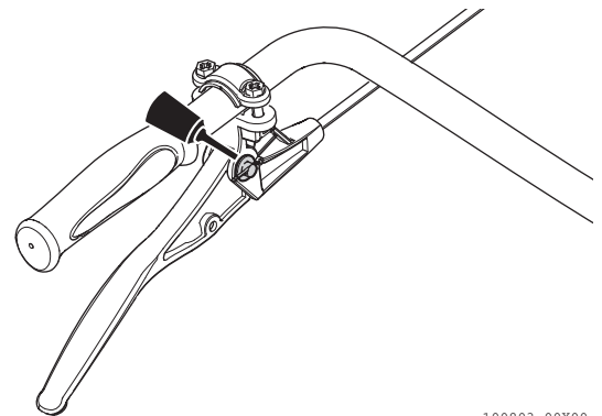
図 4-3 主クラッチレバー支点
