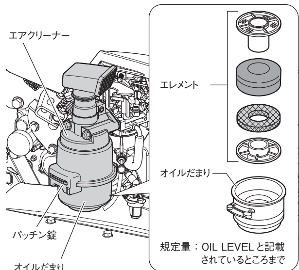
図 4-20 エアクリーナー
