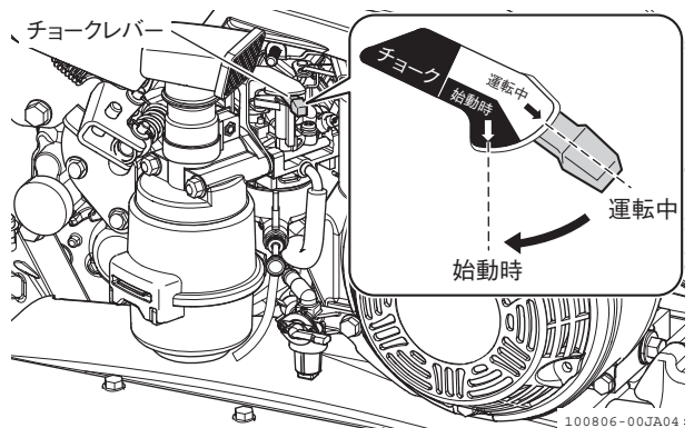
図 2-20 チョークレバー
