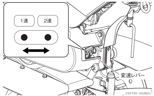
図 2-7 変速レバー (-D、-S型式)
